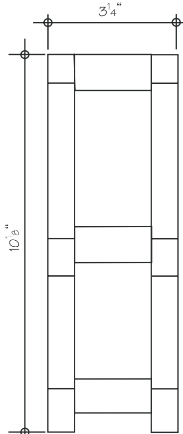
ELEVATION
